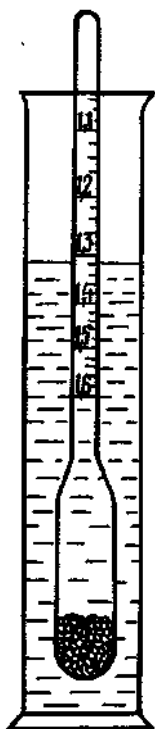
Рис. 1. Определение плотности жидкости при помощи ареометра
