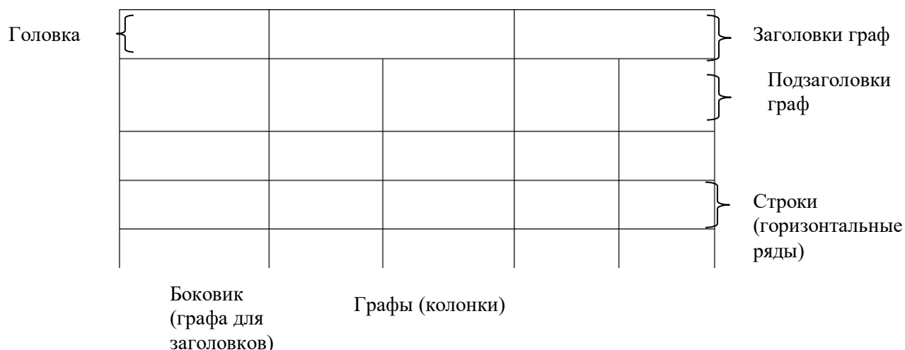
Рисунок 2 – Макет таблицы
